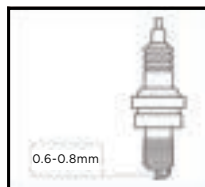
Jeu de la bougie d'allumage
